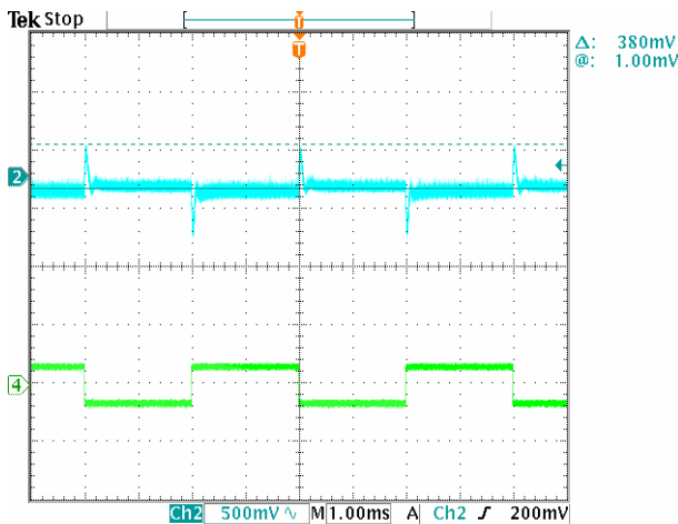
图 17. V_{in}=48v , I_{out}= 10\sim 30A , 2.5A/\mu s 动态负载下, 输出电压的动态范围。波形 2 是动态负载下的动态响应, 波形 4 是负载电流( 2.5A/\mu s ), 输出电容负载为 10\mu F 。
