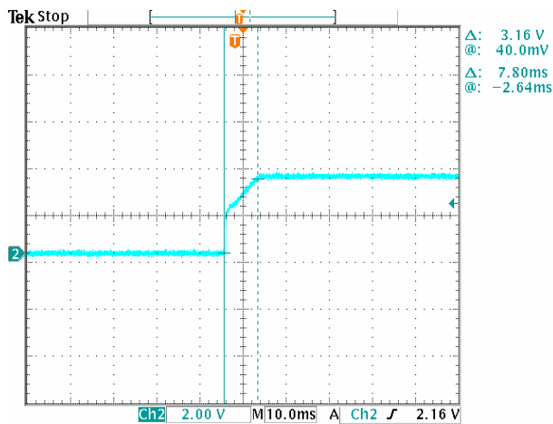
图 19. V_{in}=48v , I_{out} = 0A 时的输出电压过调与上升时间, 输出电容负载为 100\mu F , 开/关管脚有效以开启此单元。
