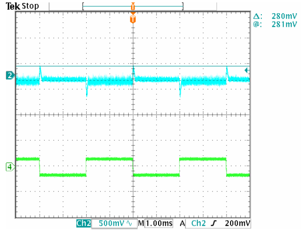
V_{in}=48v , I_{out}= 10\sim 30A , 2.5A/\mu s 动态负载下, 输出电压的动态响应。波形 2 是动态负载下的动态响应, 波形 4 是负载电流( 2.5A/\mu s ), 输出电容负载为 2200\mu F 。
