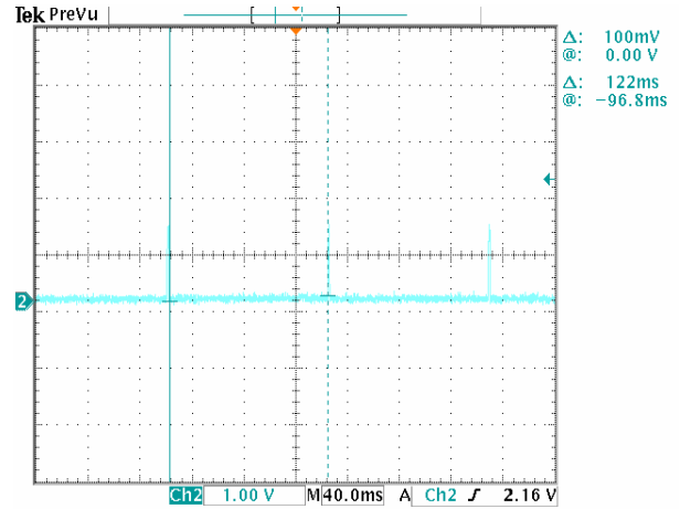
图 22. 在 10m\Omega 短路与 48Vin 下重启时的短路保护条件的输出波形
