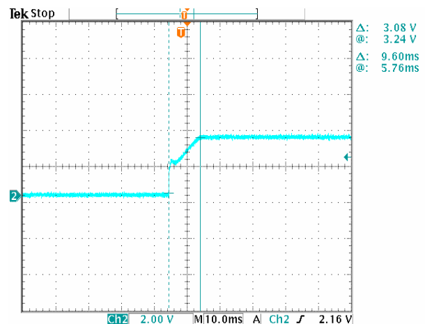
图20. V_{in}=48v , I_{out}=20A 时的输出电压过调与上升时间, 输出电容负载为 100\mu F , 开/关管脚有效以开启此单元。
