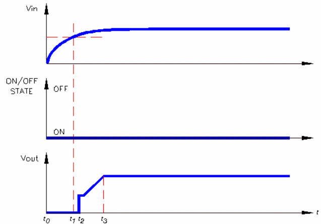
图 10 开启波形
