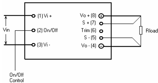
图 1: 逻辑开/关功能的典型电路
