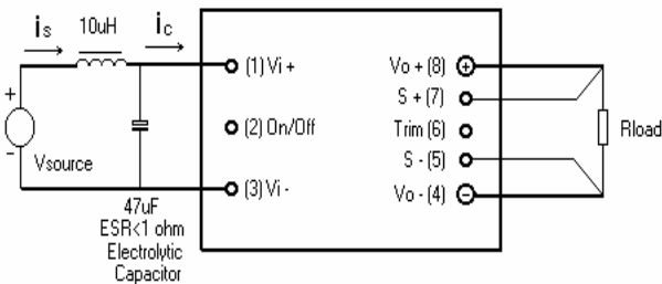
图 29. 为测量输入反射纹波电流 i_c 和 i_s 进行的测试。
