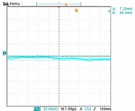
图 28. 输入电感为 10uH 时，输入反射纹波电流与波形的关系， V_{in}=48v , i_{out}=40A 。
