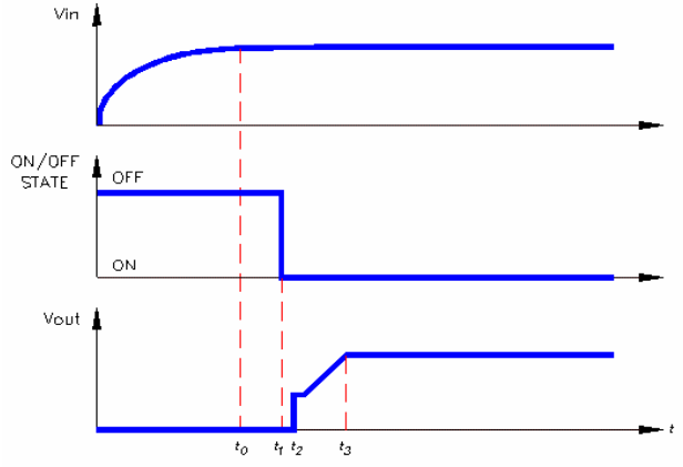
图 11. 运用开/关管脚开启
