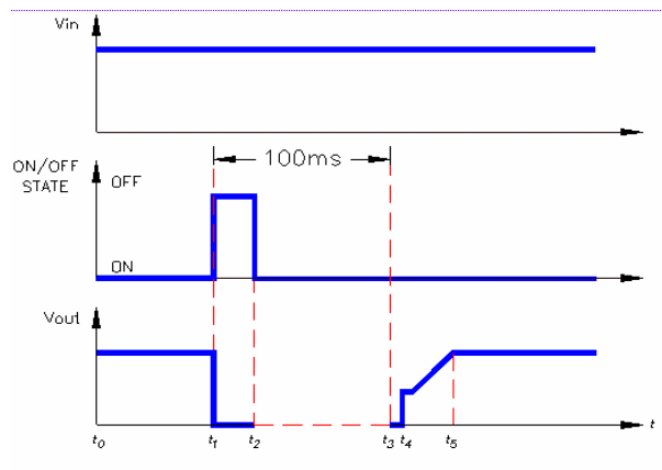
图 12. 使用开/关管脚关闭并重启
