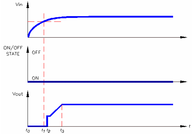
图 10 开启波形
