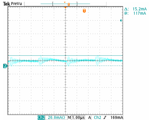
图 27. 不带输入电感的输入反射波纹电流与波形的关系。Vin=48v, Iout=40A, 100ma/Div (50mv/div 的电流探头)
