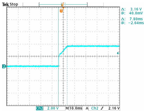
图 19. Vin=48v, Iout = 0A 时的输出电压过调与上升时间, 输出电容负载为 100uF, 开/关管脚有效以开启此单元。
