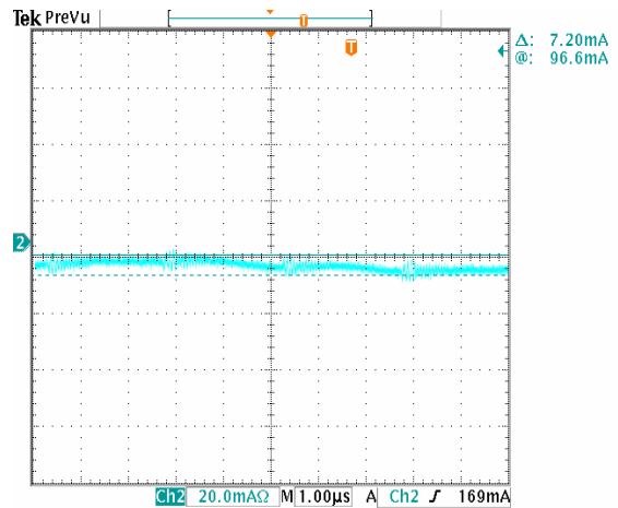
图 28. 输入电感为 10uH 时，输入反射波纹电流与波形的关系，Vin=48v, Iout=40A。
