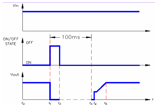
图 12. 使用开/关管脚关闭并重启
