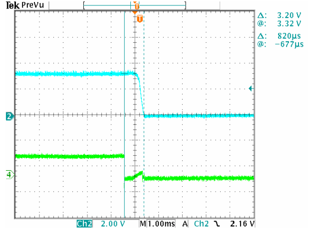
图 14. 关闭时间与输入开/关管脚的关系。波形 2 为输出电压，波形 4 为正开/关逻辑信号。输入电压为 48V，输出电流为 20A，输出电容负载为 100uf。
