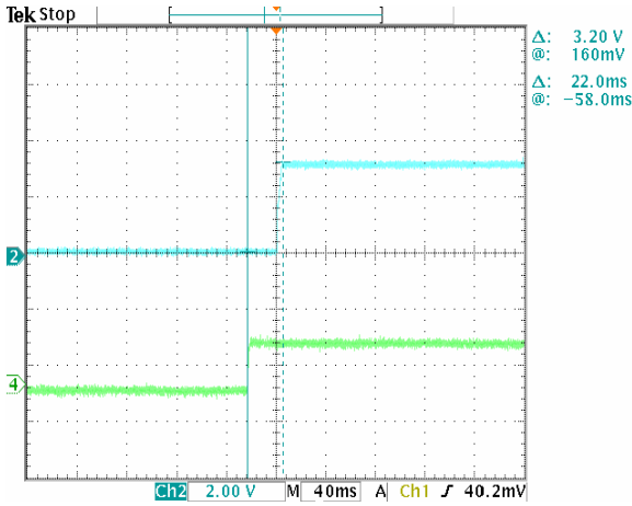
图 13. 开启时间与输入开/关管脚的关系。波形 2 为输出电压，波形 4 为正开/关逻辑信号。输入电压为 48V，输出电流为 20A，输出电容负载为 100uf。
