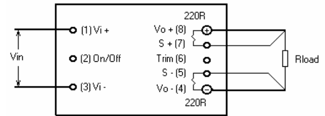
图 2: 遥感电路
