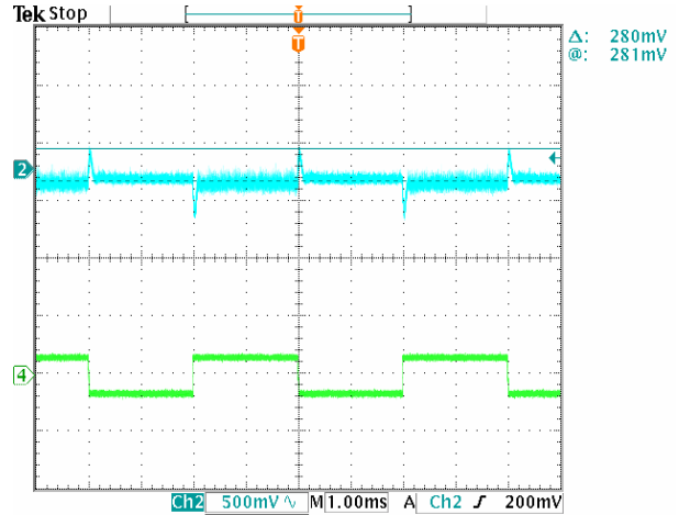
Vin=48v , Iout= 10~30A, 2.5A/us 动态负载下, 输出电压的动态响应。波形 2 是动态负载下的动态响应, 波形 4 是负载电流(2.5A/us), 输出电容负载为 2200uF。
