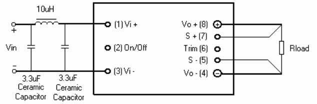
图 7. EMC 的外部滤波器
