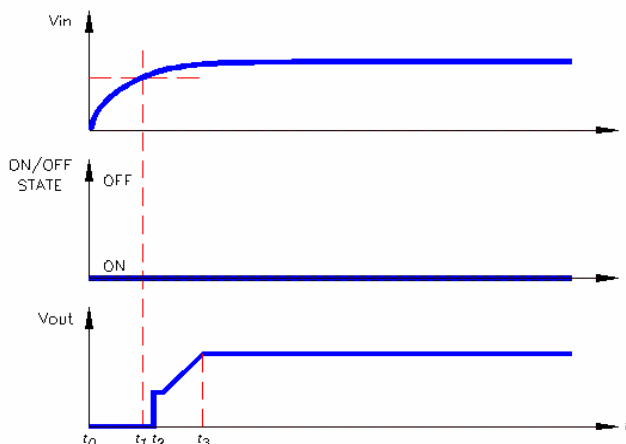
图 10 开启波形
